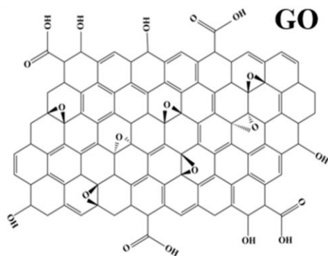
Rys. 1. Przykładowa struktura tlenku grafenu 3
